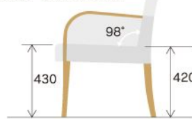
通常の肘付椅子 (W390-41N5)
