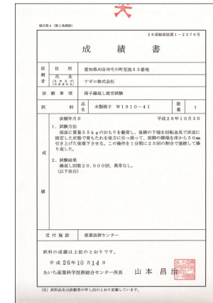
成績書 あいち産業科学技術センター 繰り返し回数 20,000回 異常なし
