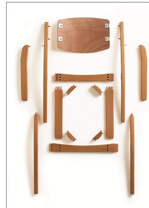
解体フレームパネル ※W1910と同一フレームを使用
